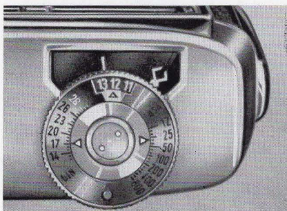
Belichtungsmesser mit Nachführsystem
